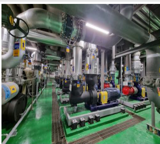
고효율 냉동 System 교체(ESCO) 사업 추진 ( '22년~)
